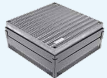
Rejilla para terraza TR-H 40 x 40-95 con pieza de elevación y con tapa elevada
